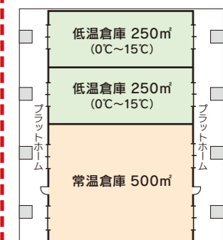
CFS倉庫の平面図▶
